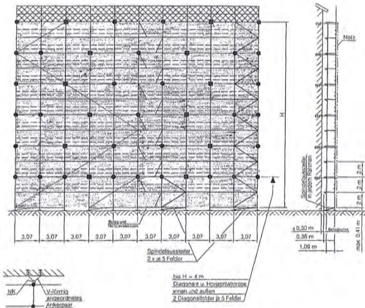
Detail Verankerung
