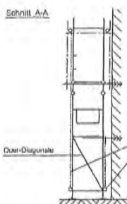
Schnitt A-A
