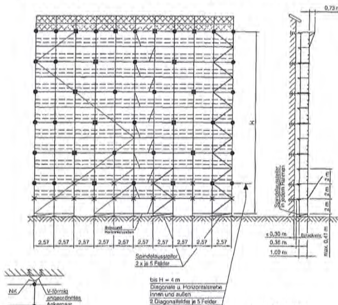
Detail Verankerung
