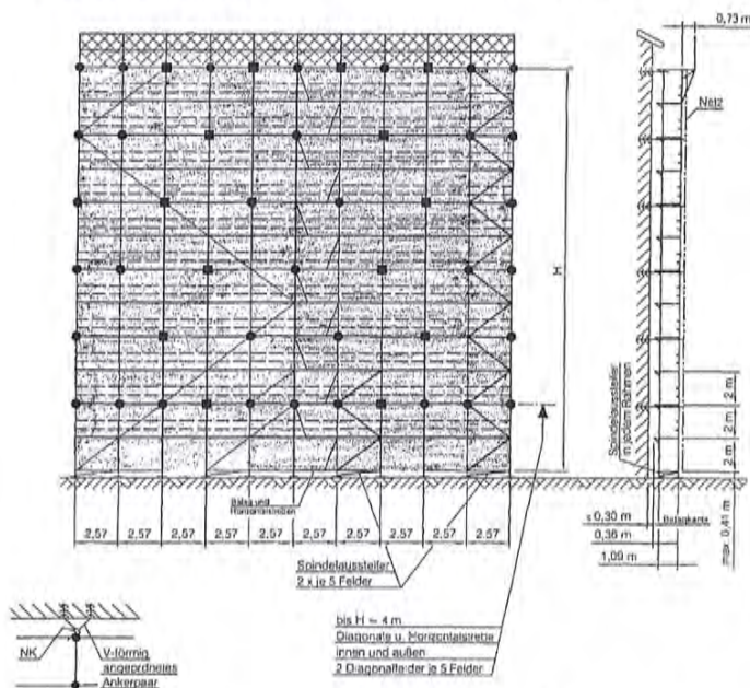
Detail Verankerung
