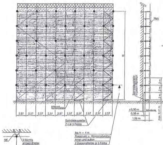
Detail Vorankerung
