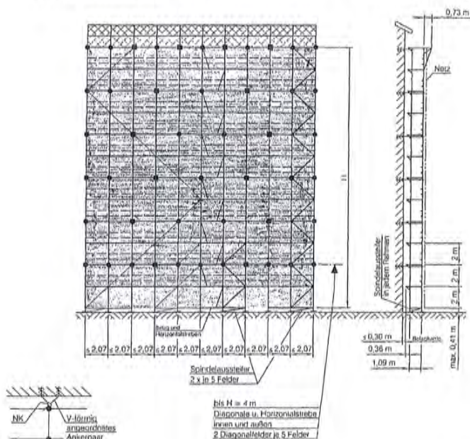
Detail Verankerung
