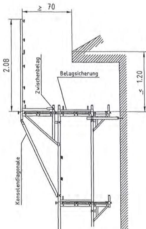
Verankerungsbeispiele
