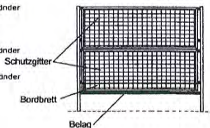
mit Schutzgittern
