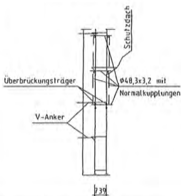
Schnitt A-A
