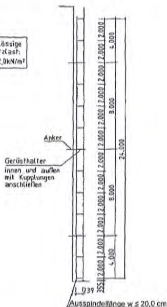
Schnitt A-A
