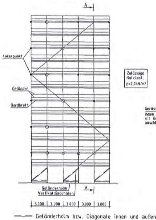
Ansicht
