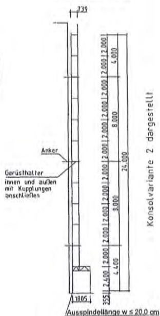
Schnitt A-A
