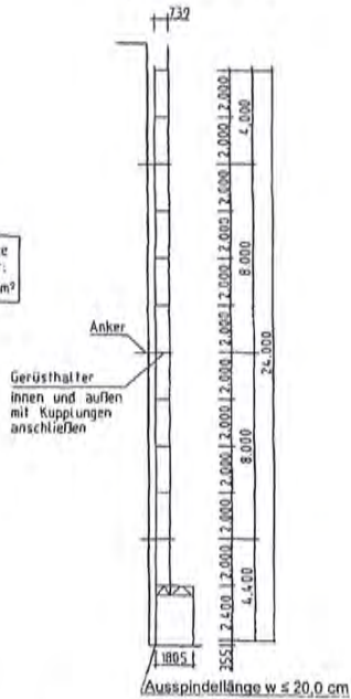
Schnitt A-A
