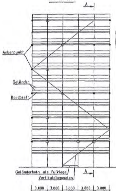
Ansicht
