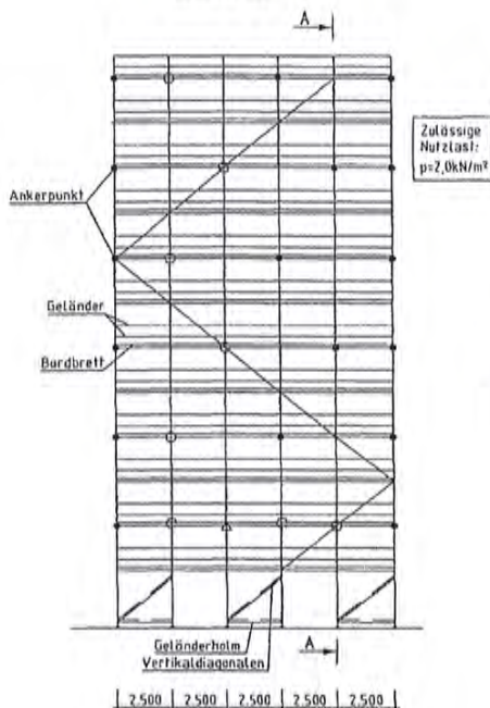
Ansicht
