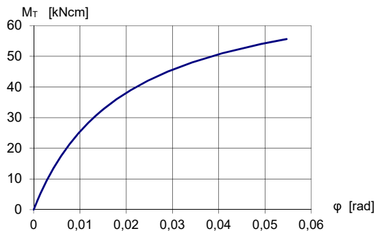
Bild 4: Drehfedersteifigkeit im Rohrriegelanschluss bei Torsionsmoment um die Riegelachse
