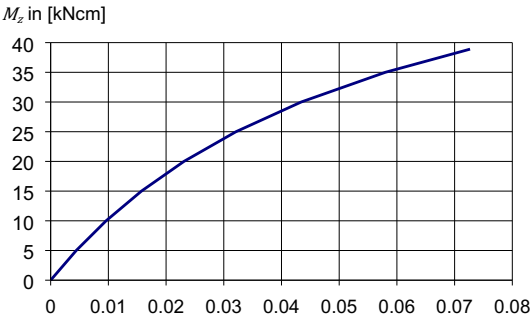
Bild 7: Drehfedersteifigkeit bezüglich M_z in der Keilkopfkupplung doppelt nach Anlage A, Seite 72 und der Doppelkeilkopfkupplung nach Anlage A, Seite 71
