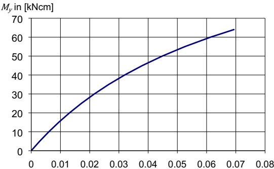
Bild 6: Drehfedersteifigkeit bezüglich M_y der Doppelkeilkopfkupplung nach Anlage B, Seite 71 entsprechend des Ersatzmodells nach Anlage A, Seite 5
