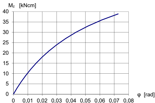
Bild 3: Drehfedersteifigkeit im Rohr- und U-Riegel anschluss bei Biegung in der horizontalen Ebene
