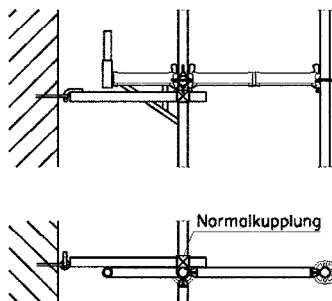
Bild D.2b: Gerüsthälter
