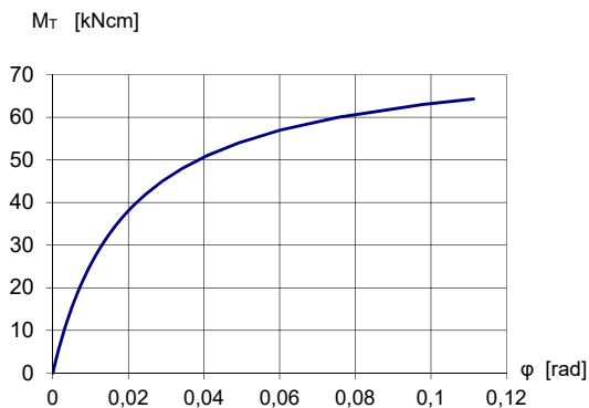
Bild 4: Drehfedersteifigkeit im Rohrriegelanschluss bei Torsionsmoment um die Riegelachse
