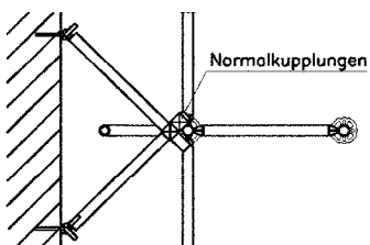
Bild D.2c: V-Halter
