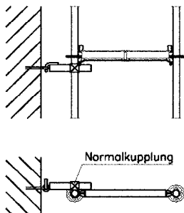
Bild D.2a: Gerüsthälter
