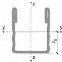
Bild 2: Kennwerte des U-Profils 53 ohne Lochung
