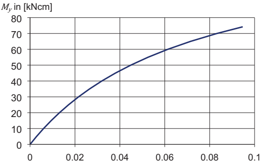
Bild 6: Drehfedersteifigkeit bezüglich M_y der Doppelkeilkopfkupplung nach Anlage B, Seite 03.13.00 entsprechend des Ersatzmodells nach Anlage A, Seite 5
