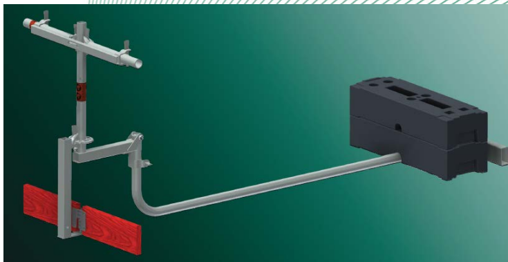
Bild 3: Komponenten des Seitenschutzsystems
