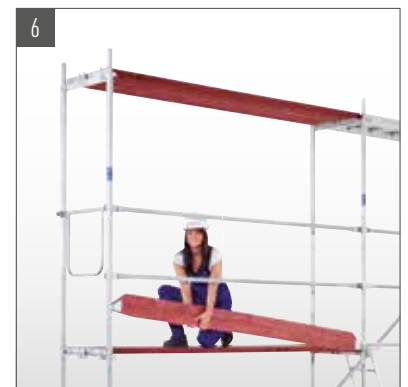
6 Vertikalrahmen und Beläge der nächsten Lage montieren, Diagonale, Geländer und Bordbretter einhängen.
