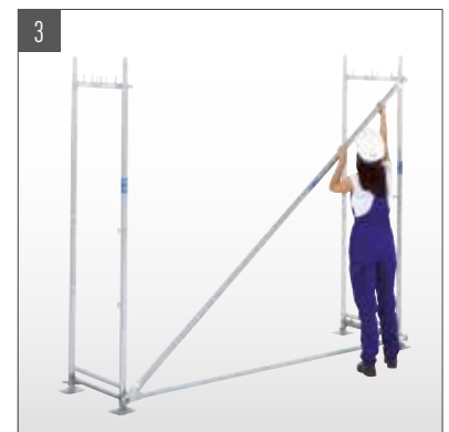
3 Diagonale über Kippstifte montieren.
