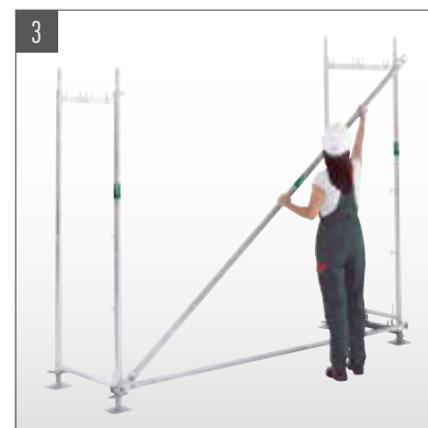
3 Diagonale über Kippstifte montieren.
